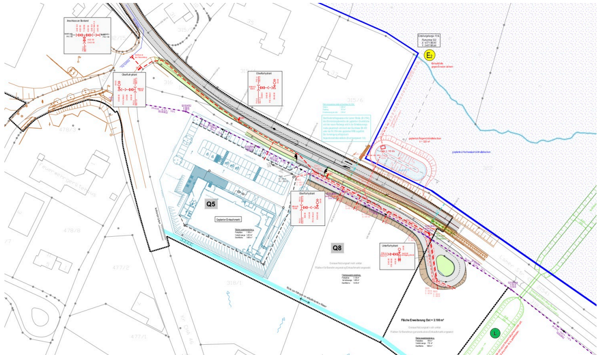
Planausschnitt Niederschlagswasserkonzept, EBB Ingenieurgesellschaft mbH
